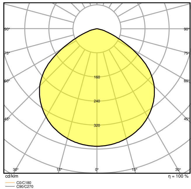
HB-DALI-155W-4000K-110DEG-IP65
