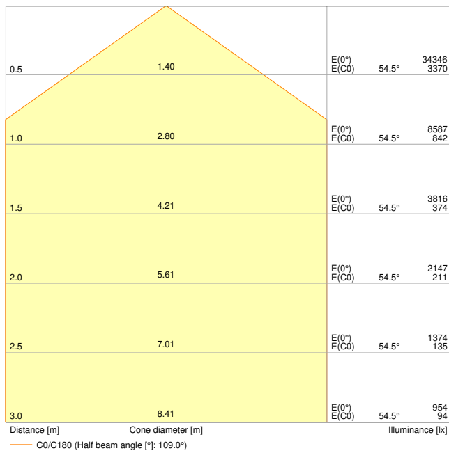
HB-DALI-155W-4000K-110DEG-IP65
